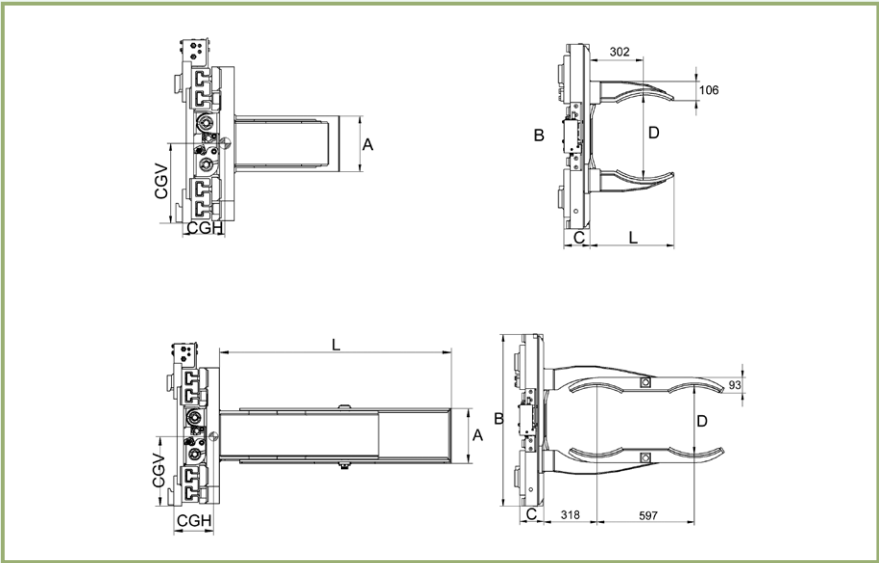
非侧移式 Non-Sideshifting
